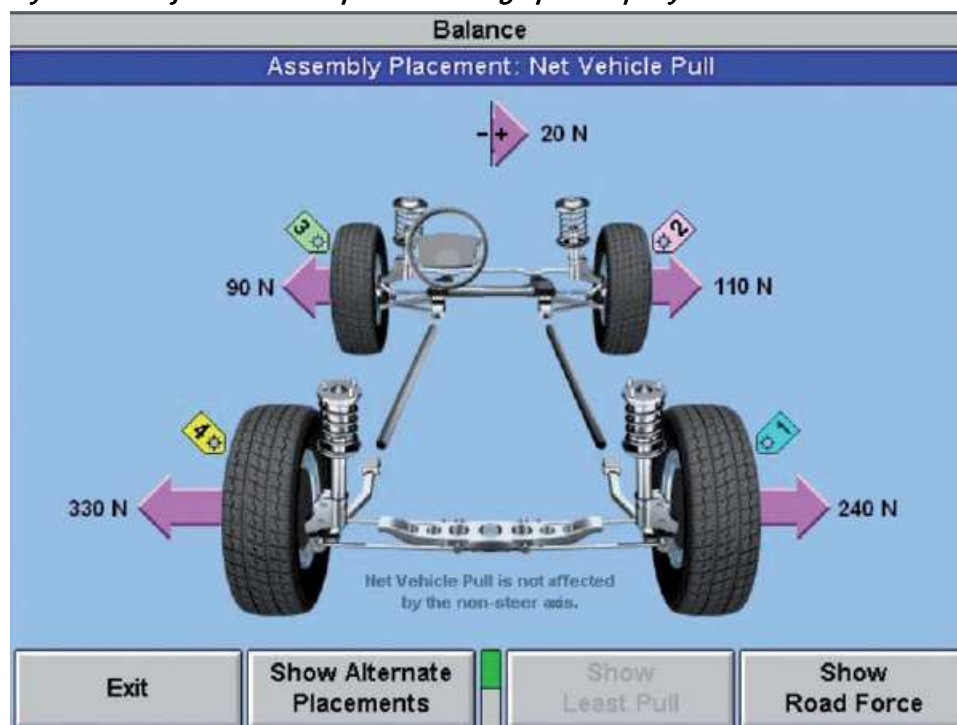
Rys.: Przykładowy rozkład sił przy zamianie kół miejscami
