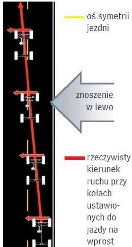
Rys.: Ściąganie samochodu pod wpływem bocznej siły znoszącej
